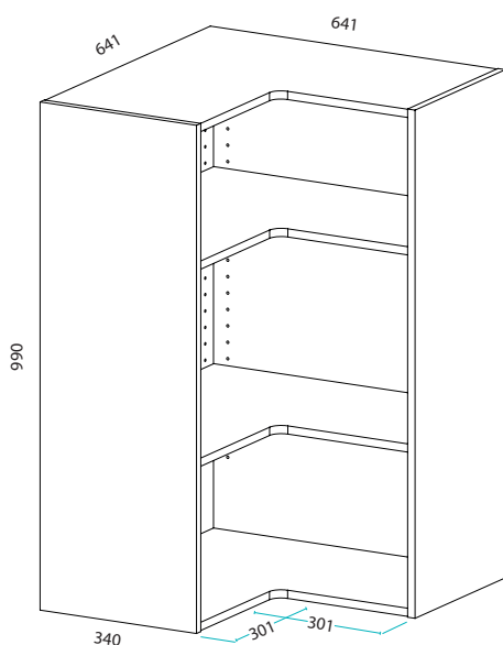
Oven leveys 2 x 275 mm
