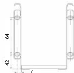
Etusarjan kiinnike
